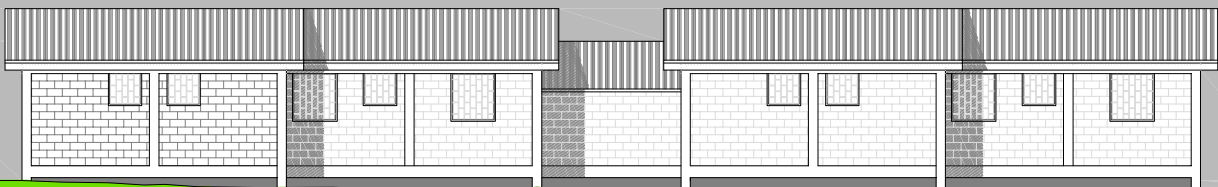
ALZADO LATERAL. E:1/200
